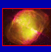
M27 / NGC6853
